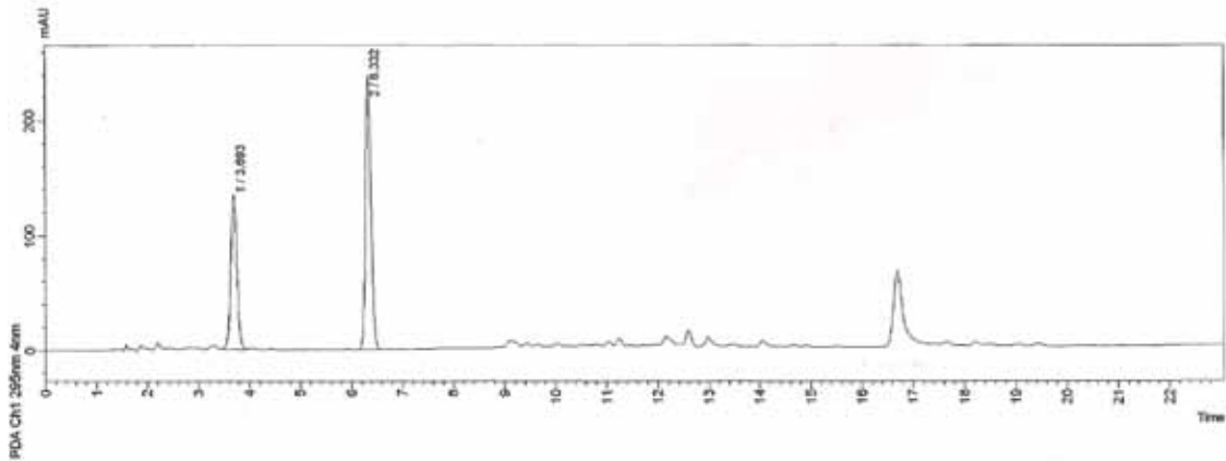
Fig. 8: Cromatograma de la fracción de cascarósidos obtenidos por TLC.
