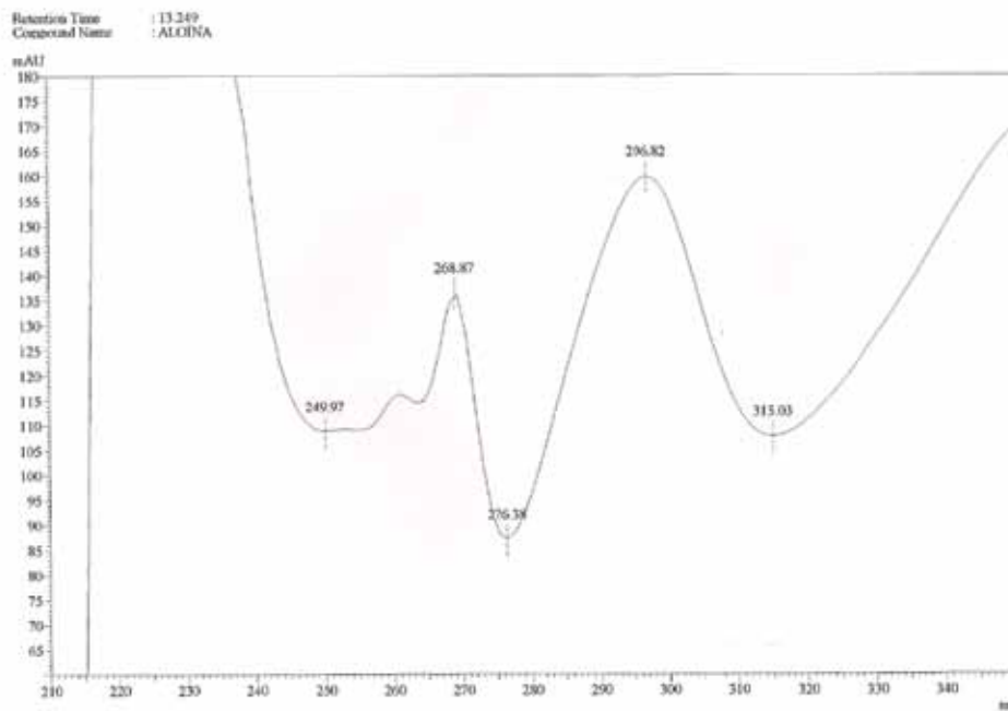
Fig. 18: Espectro el pico correspondiente a aloína testigo de T_R = 13.249 .
