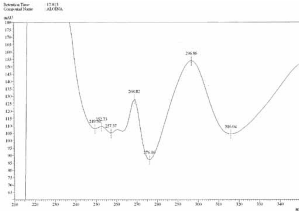
Fig. 17: Espectro del pico correspondiente a aloína de T_R = 12.813 en la muestra en el extracto de aloe.
