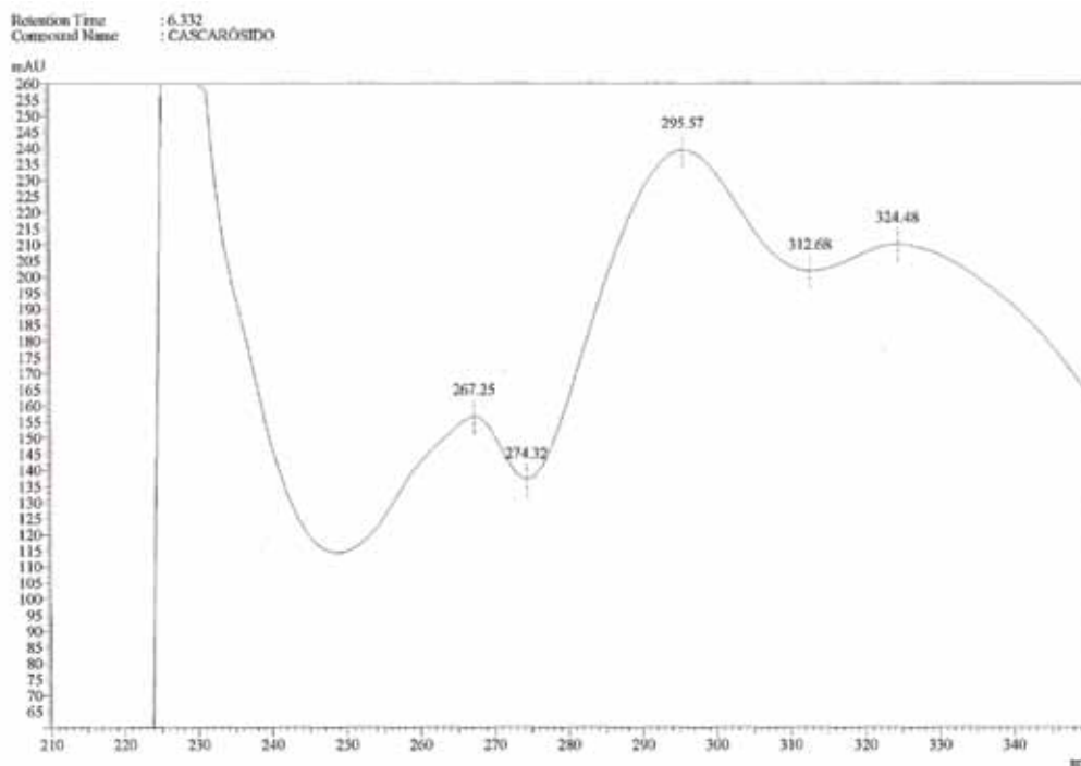
Fig. 10: Espectro Cascarósido (Tr = 6.332min).
