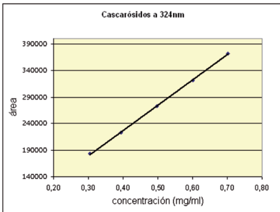
Fig. 15: Linealidad del método para Cáscara Sagrada. R 2 = 0,9992.
