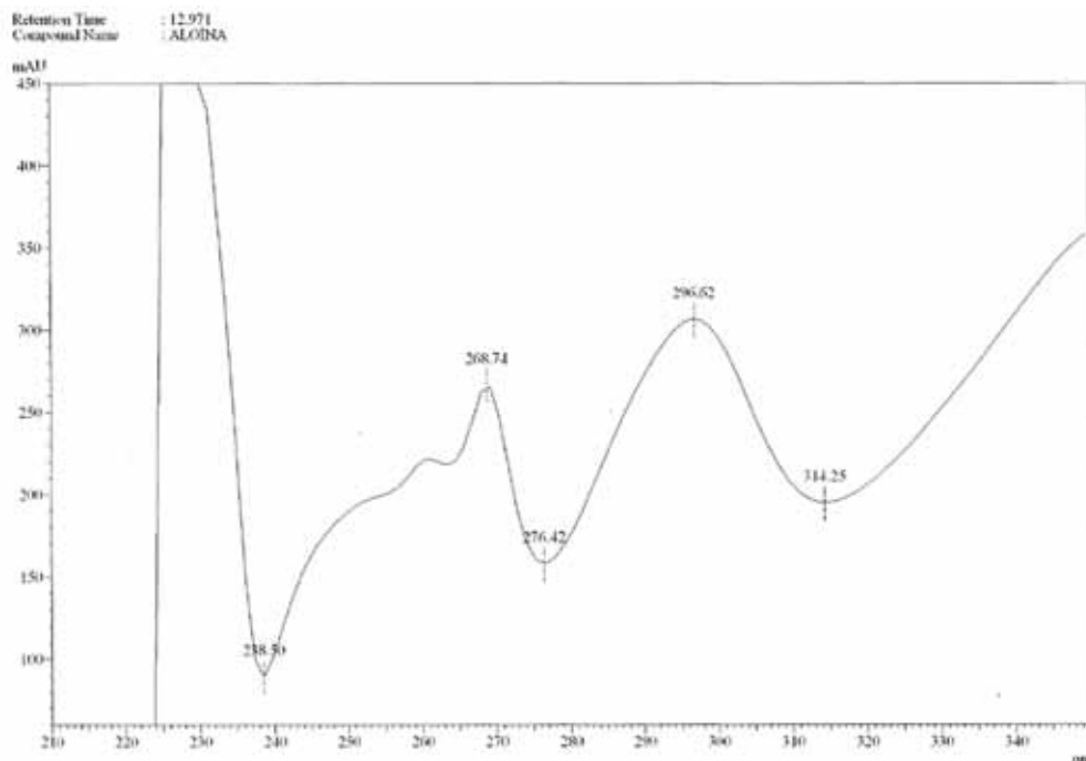
Fig. 12: Espectro de aloina A/B.
