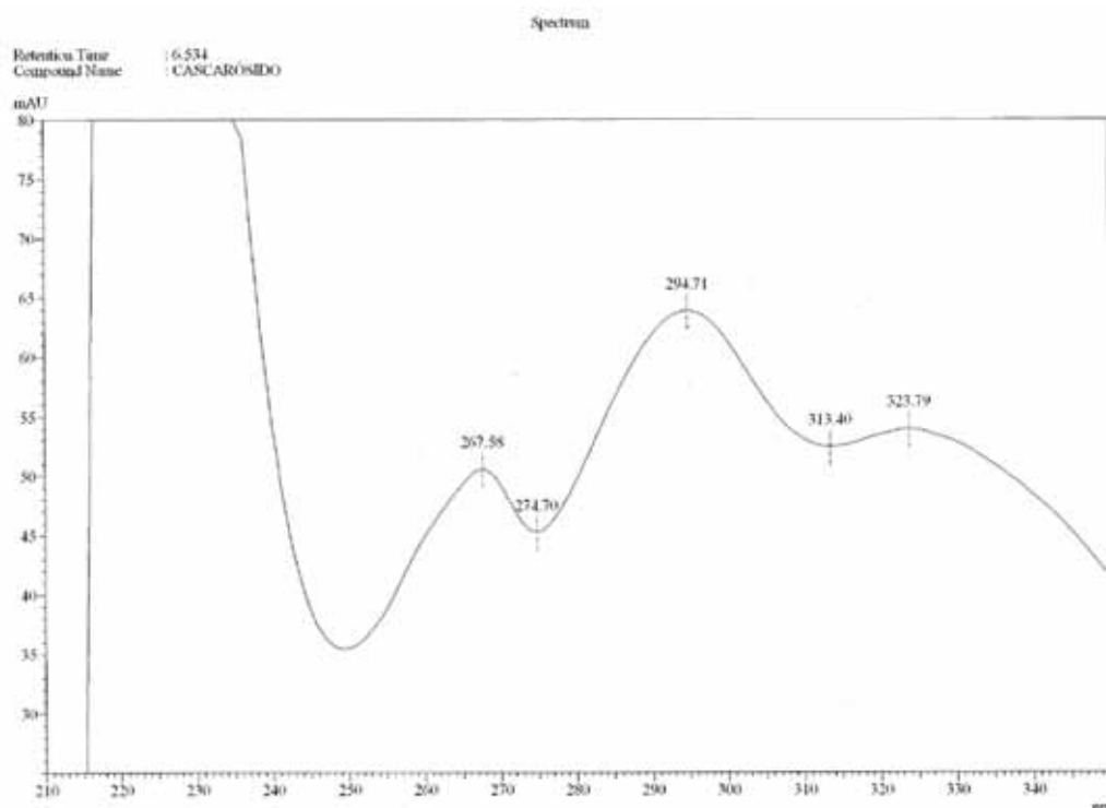
Fig. 14: Espectro del pico correspondiente al cascarósido de Tr = 6.534min en el cromatograma del extracto de Cáscara Sagrada.
