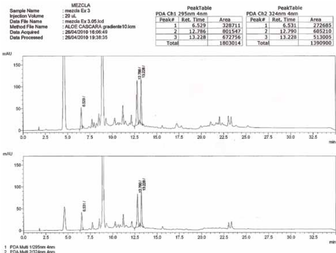
Fig. 22: Cromatograma solución Cáscara Sagrada y Aloe (extracto 3).
