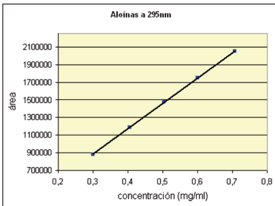
Fig. 19: Linealidad de Aloe R^2 = 0,998 .
