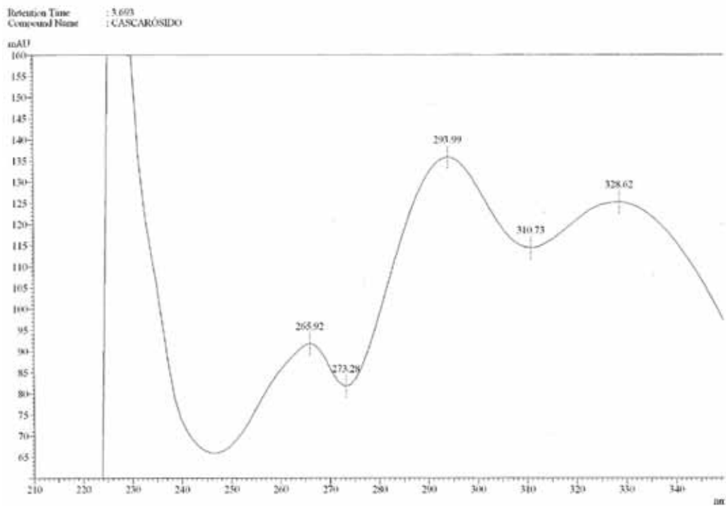
Fig. 9: Espectro Cascarósido (Tr = 3.693min).
