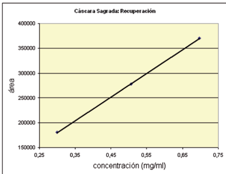
Fig. 20: Linealidad de recuperación de Cáscara Sagrada.
