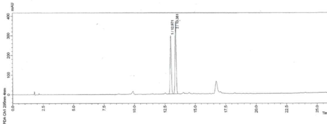
Fig. 11: Cromatograma Aloínas A/B.
