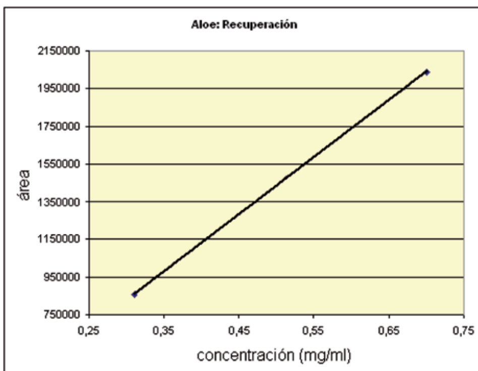
Fig. 21: Linealidad de recuperación de Aloe.
