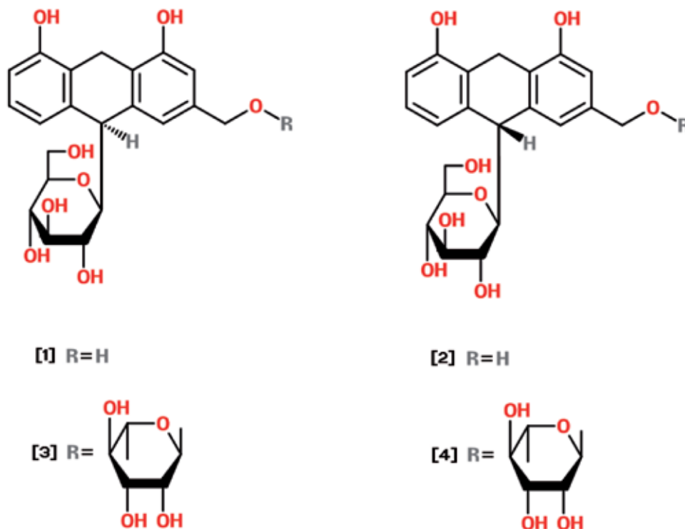
Fig. 2: [1] Aloína A ; [2] Aloína B ; [3] Aloinósido C ; [4] Aloinósido D. WHO (1999).
